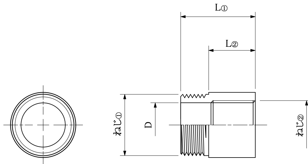
寸法表: (mm)
