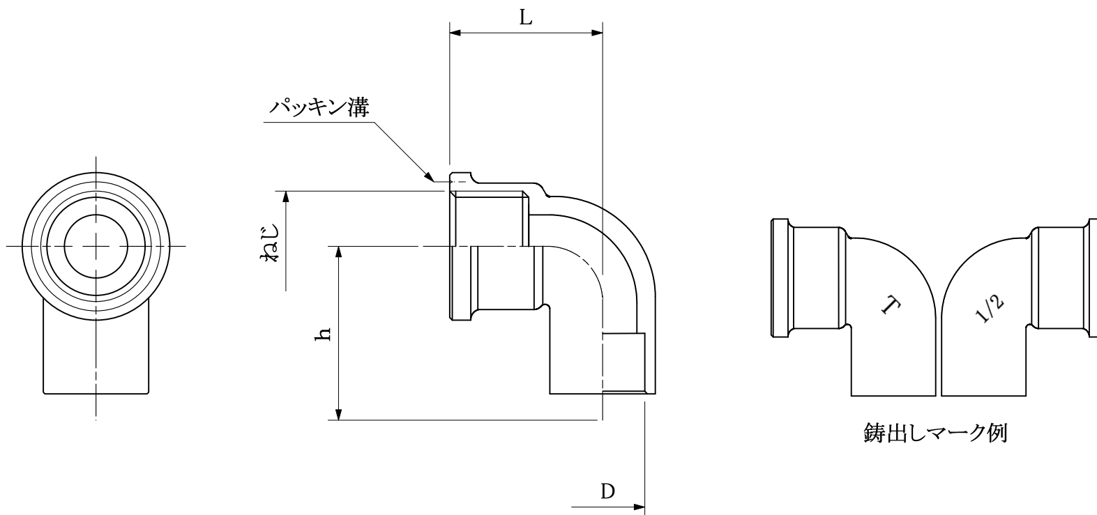
寸法表: (mm)
