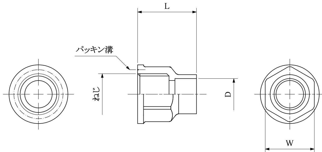
寸法表: (mm)
