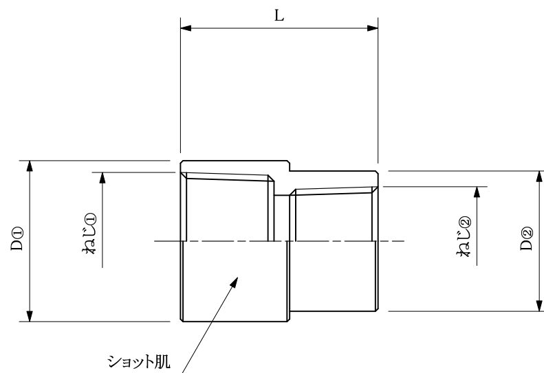
寸法表 (mm)
