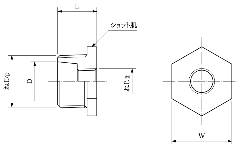
呼径25:寸法表 (mm)
