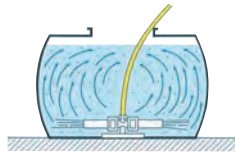
ローリータンク内の噴流(参考図)
